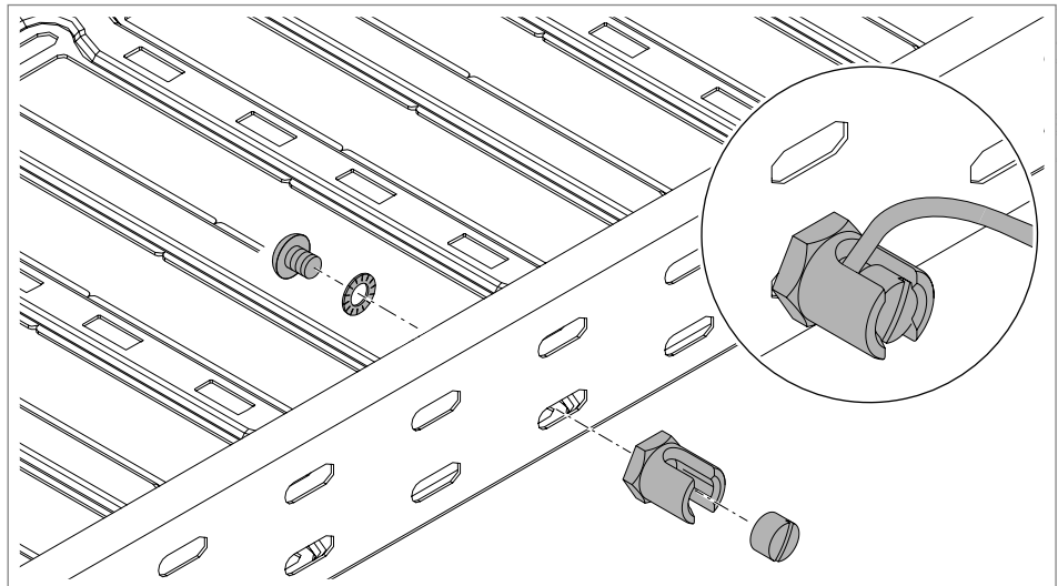
82 pav. Įžeminimo gnybto montavimas
