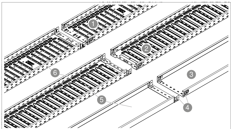
1 pav. Perforuotieji ir neperforuotieji loviai
