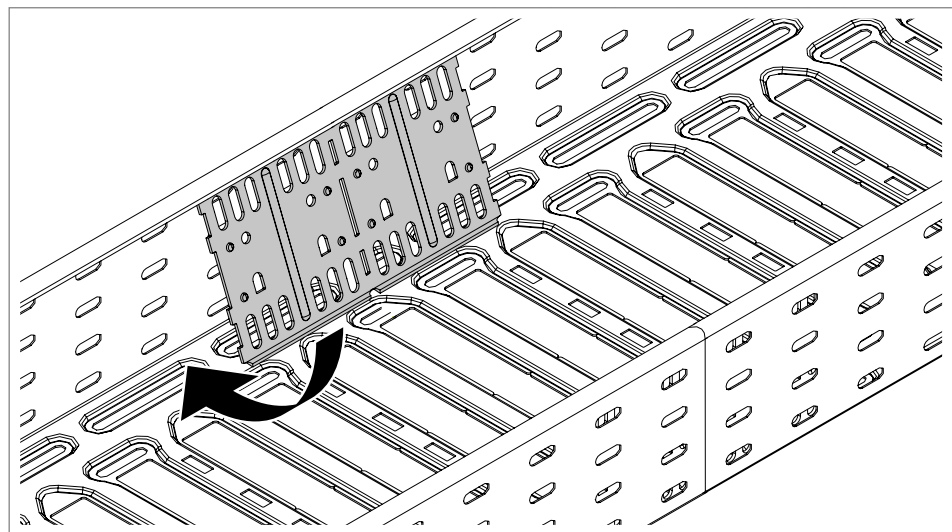
28 pav. Išilginio sujungimo elemento RLVL įstatymas
