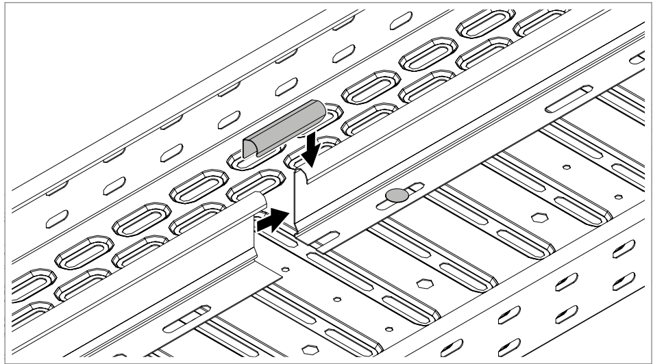
81 pav. Pertvarų sujungimas
